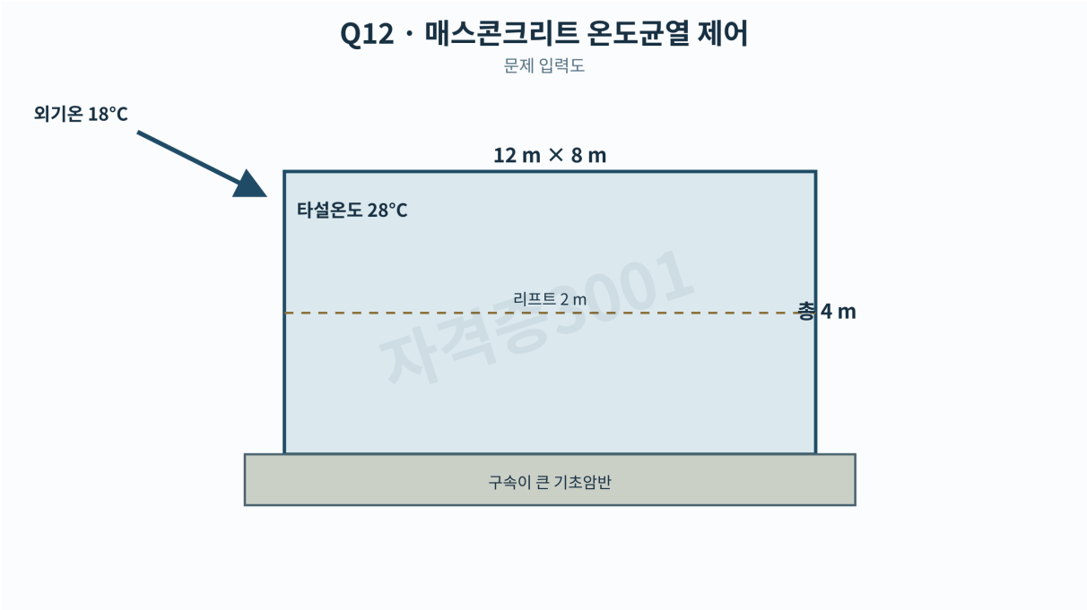
매스콘크리트 블록 치수와 타설온도·외기온·리프트 조건만 표시한 문제도
