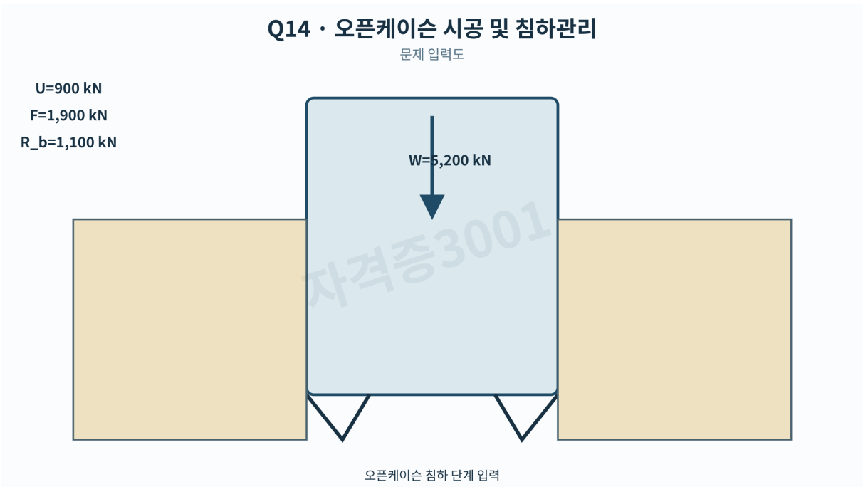
오픈케이스의 치수와 자중·부력·주면마찰·선단저항 입력만 표시한 문제도
