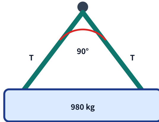
2-leg wire rope sling
