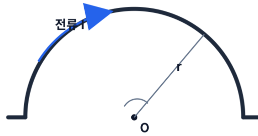
반원 중심에서의 자계 조건
