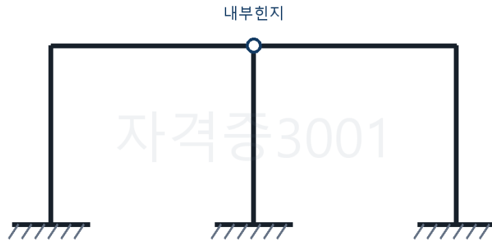
3개 고정단을 가진 2경간 골조
