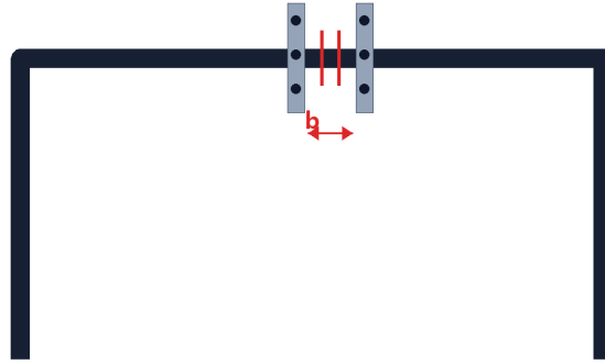
22번 포털 프레임 현장접합 상세 (자체 재작도)
