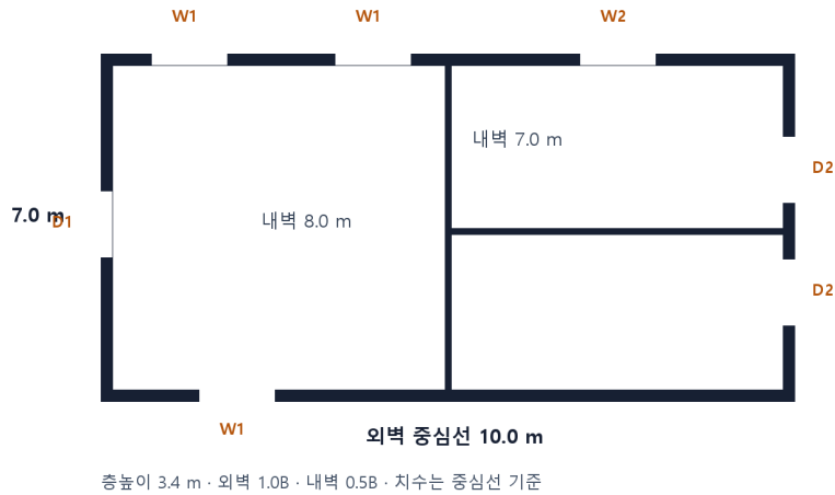
9번 적산용 평면도 (자체 제작도)
