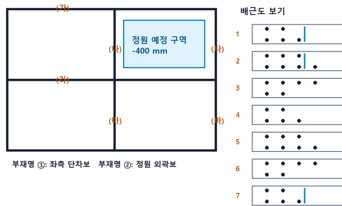
7번 옥상조경 단차부 구조평면 및 배근 보기 (자체 제작도)
