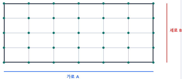
14번 경량철골천장 인서트 간격 (자격증3001 자체 재작도)
