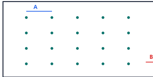
18번 슈미트해머 타격 위치 (자격증3001 자체 재작도)
